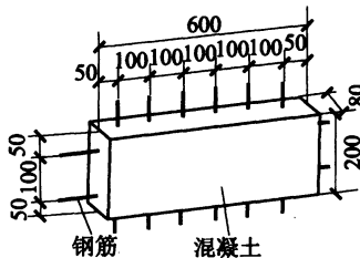
图 9 试样的构造和尺寸
