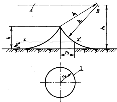
图 D.0.1 单支接闪器的保护范围
