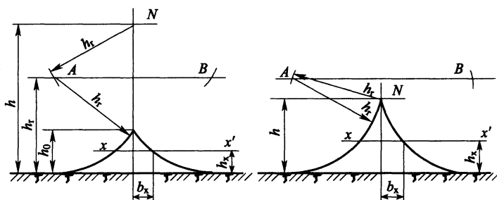
(a) 当 h 小于 2h_r , 且大于 h_r 时
