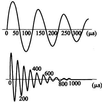
图 10 具有代表性的冲击电流波形
