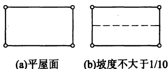
图 B.0.1 建筑物易受雷击的部位(一)
