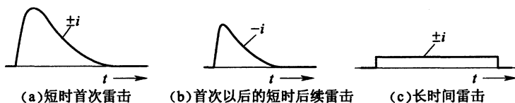
图 F.0.1-1 闪电中可能出现的三种雷击
